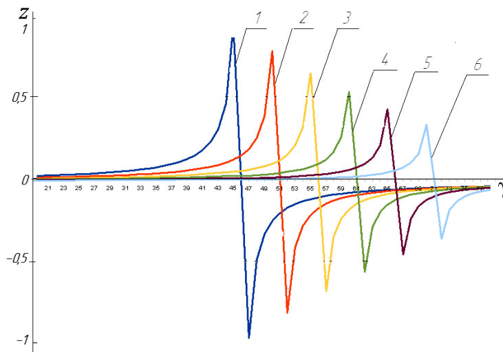
Рис.3. Залежності показника Z від кутів розкилу культиваторних лап \gamma та кутів тертя \varphi : 1 - \varphi = 0^\circ ; 2 - \varphi = 10^\circ ; 3 - \varphi = 20^\circ ; 4 - \varphi = 30^\circ ; 5 - \varphi = 40^\circ ; 6 - \varphi = 50^\circ
