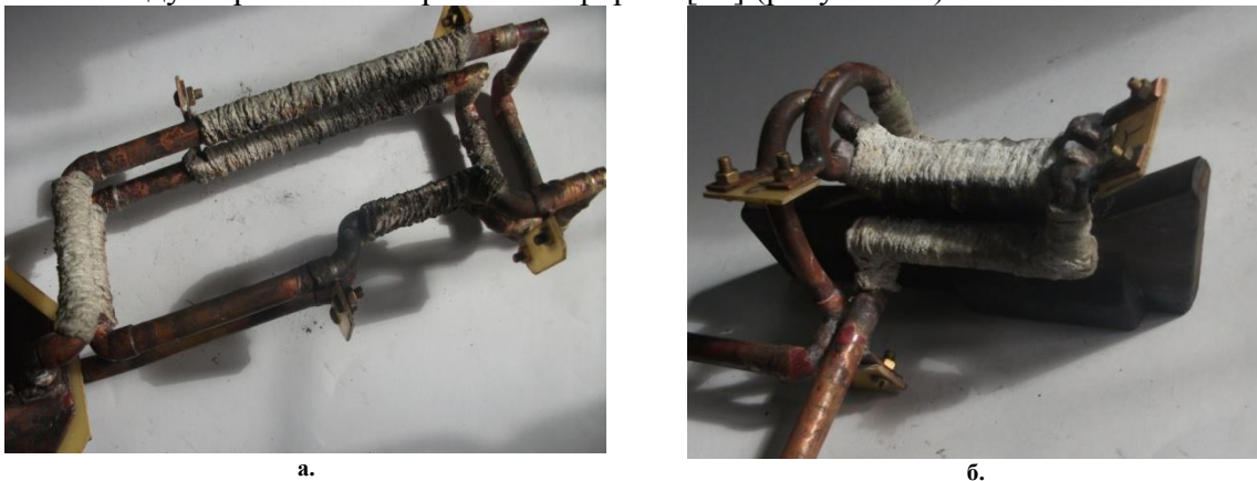
Рис. 2. Индукторы оптимизированной формы для упрочнения долота сеялки Grimera DMC-9000: а - двухпетлевой индуктор для ТВЧ-закалки, б - охватывающем щелевой индуктор для ТВЧ-наплавки и скоростного ТВЧ-борирования
