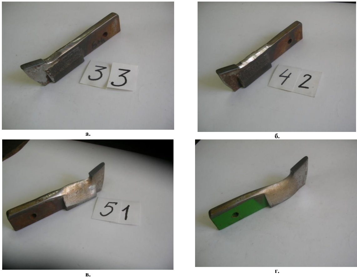
Рис. 3. Характерный износ долот сеялки Primage DMC-9000 упрочненных комбинированными покрытиями различных конструкций: а. - скоростным ТВЧ-борированием передней поверхности и ЭИН боковых поверхностей, б. - наплавкой передней поверхности сплавом ПС-14-60 и ЭИН боковых поверхностей, в. - наплавкой передней поверхности борированным сплавом ПГ-С27 и ЭИН боковых поверхностей, г. - характерный износ контрольных долот
