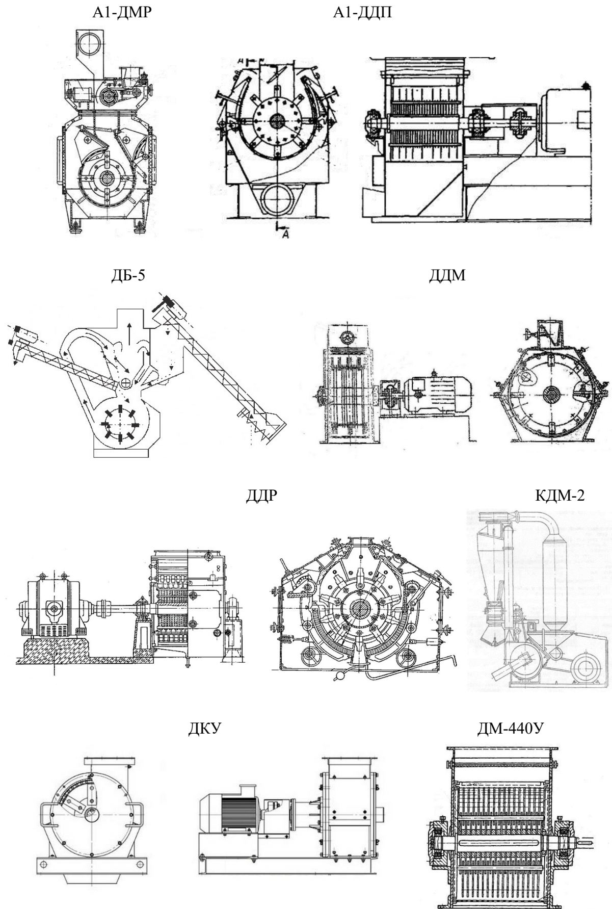
Рис. 2. Види молоткових кормодробарок.
