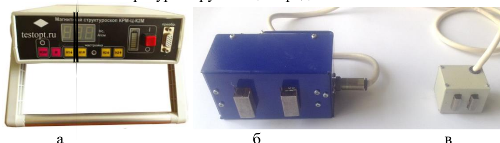
Рис.1 – Магнитный структуромер КРМ-Ц –К2М (а) с большим (б) и малым (в) магнитным преобразователем
