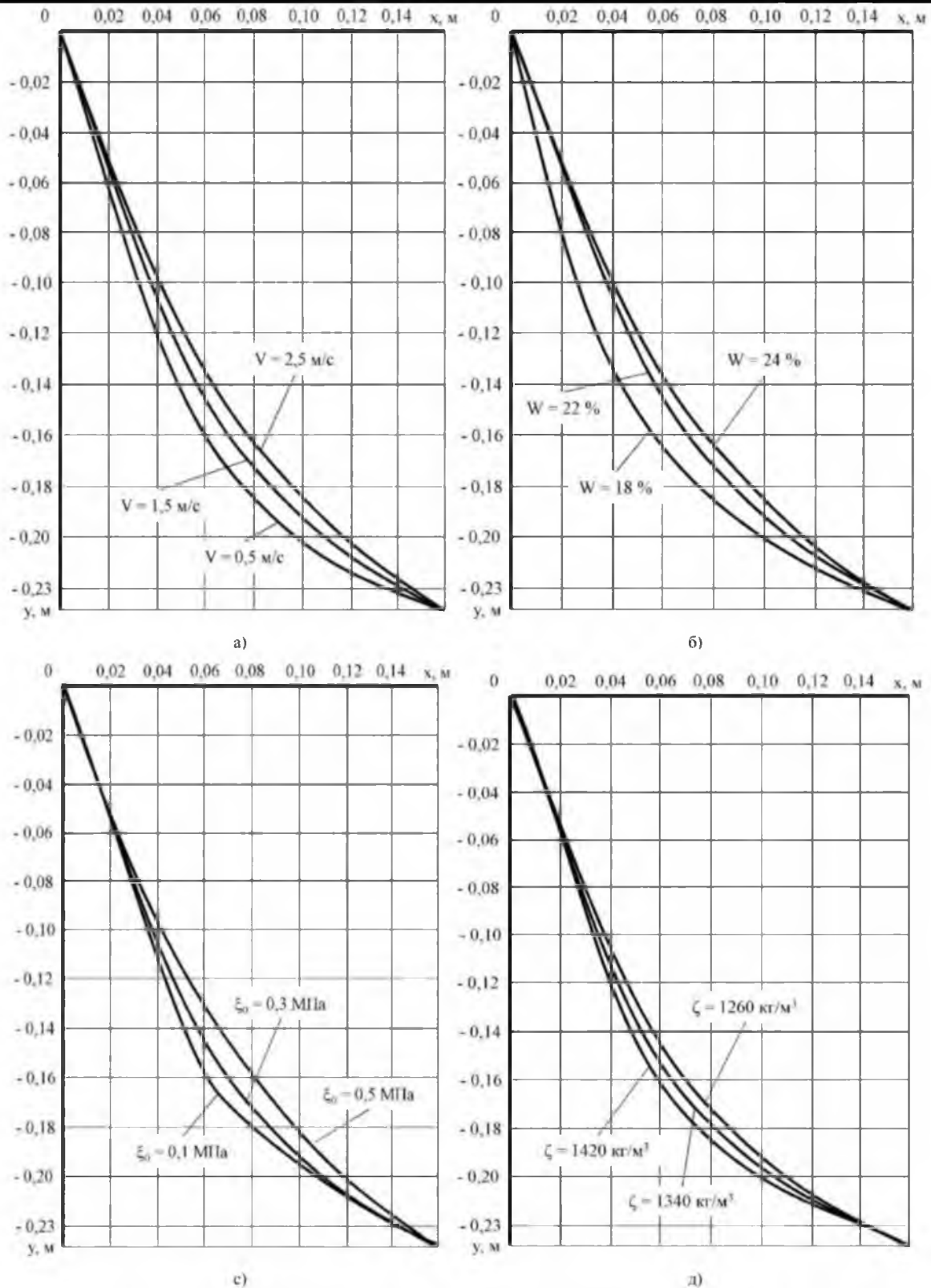
Рис.1 – Геометрична форма поверхні лани культиватора в залежності від: а) швидкості її переміщення; б) вологості ґрунту; в) коефіцієнту бокового тиску; д) щільності ґрунту
