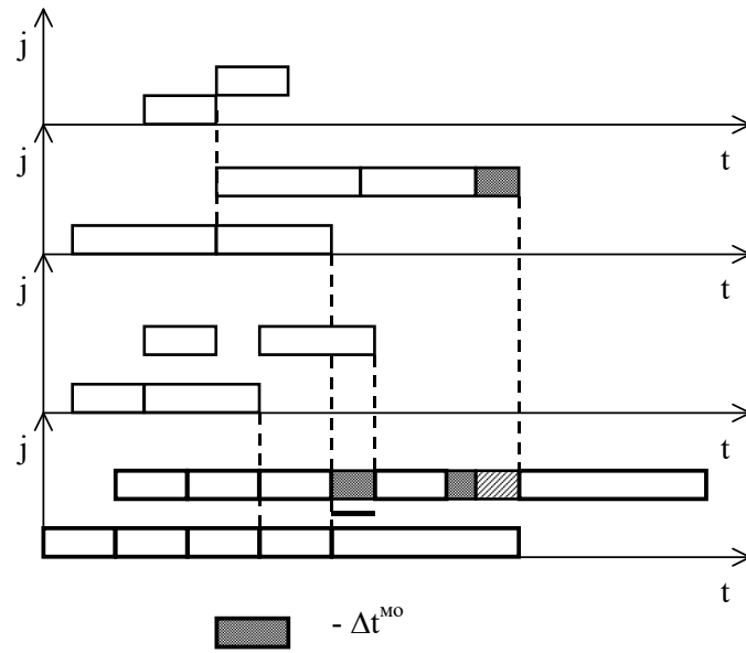
Рис.8 - Циклограма основного і рівнобіжного складання виробу по основному Аз
