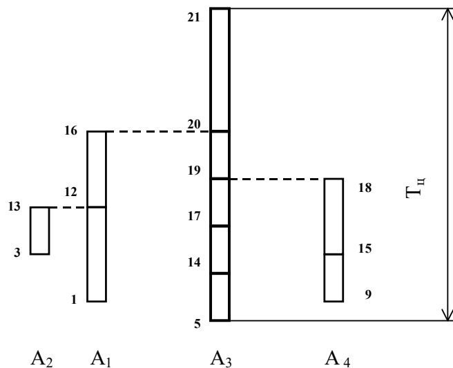
Рис.7 - Часова схема складання виробу
