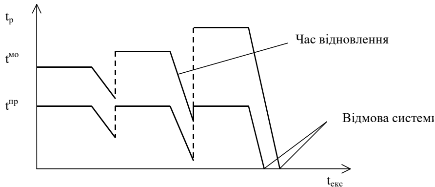
Рис.13 - Наробіток на відмову системи з резервом часу
