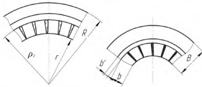
Рис.3 – Схема для розрахунку навивання смуги зі скругленими вирізами при відсутності (а) і наявності (б) неідеальної зони
